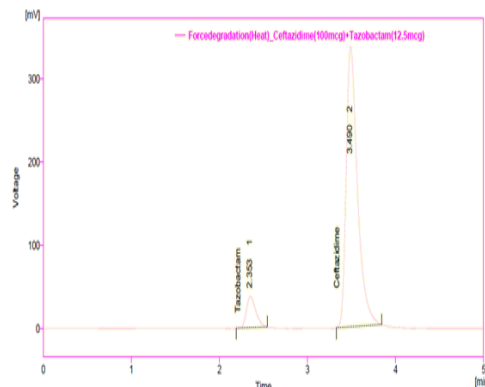
Fig: 8 Thermal Degradation
